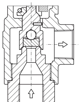
Tipo standard 240 • Standard type 240
