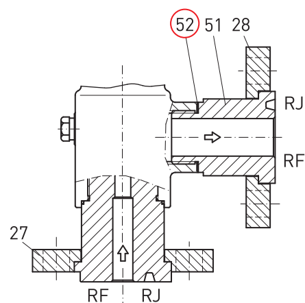
Tipo standard flangiata • Standard flanged type
