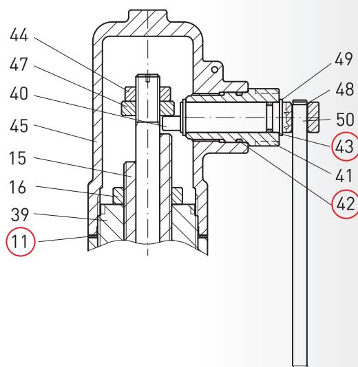
Leva di sollevamento • Lifting lever
